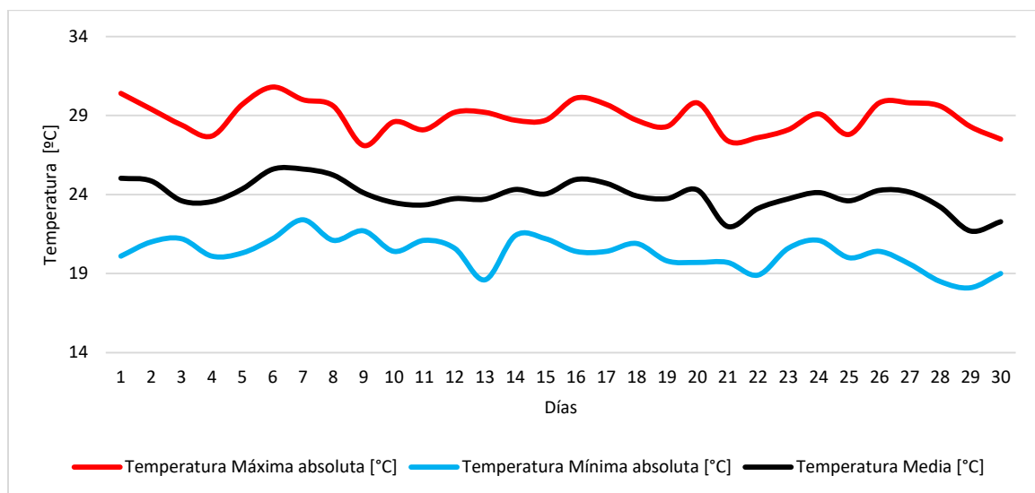
Figura 2. Temperatura del aire diaria (media, máxima y mínima). Junio de 2024
