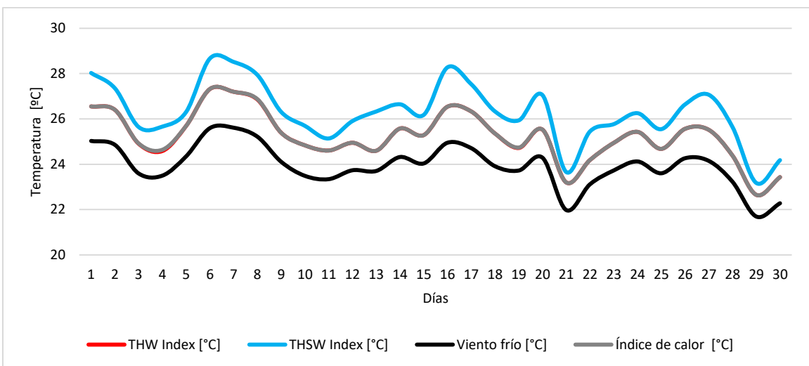
Figura 7. Índices de confort térmico. Junio de 2024
