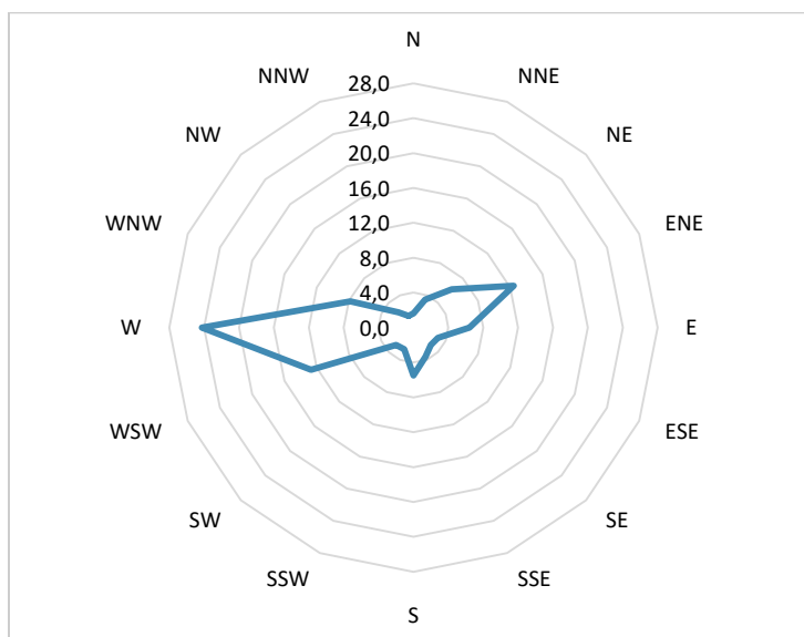
Figura 3. Dirección desde donde provienen los vientos. Junio de 2024
