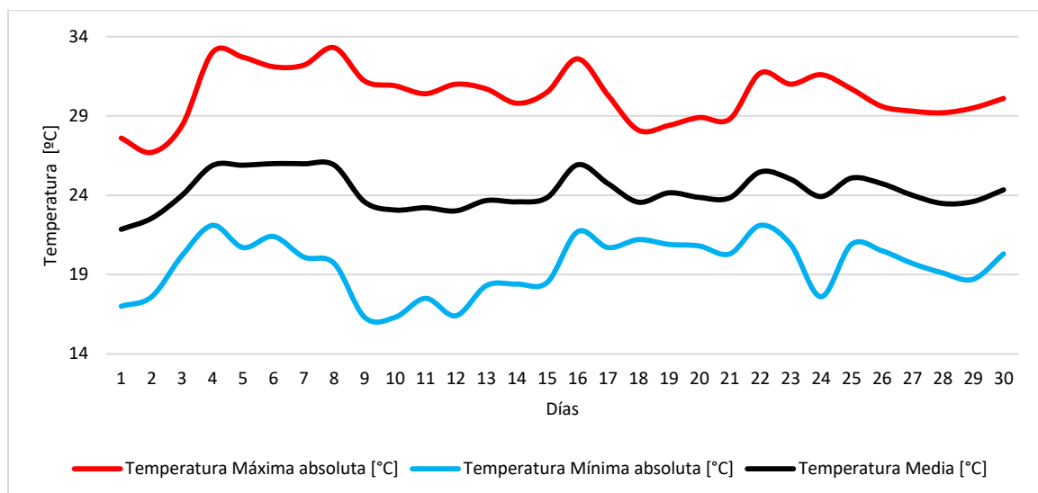
Figura 2. Temperatura del aire diaria (media, máxima y mínima). Abril de 2024
