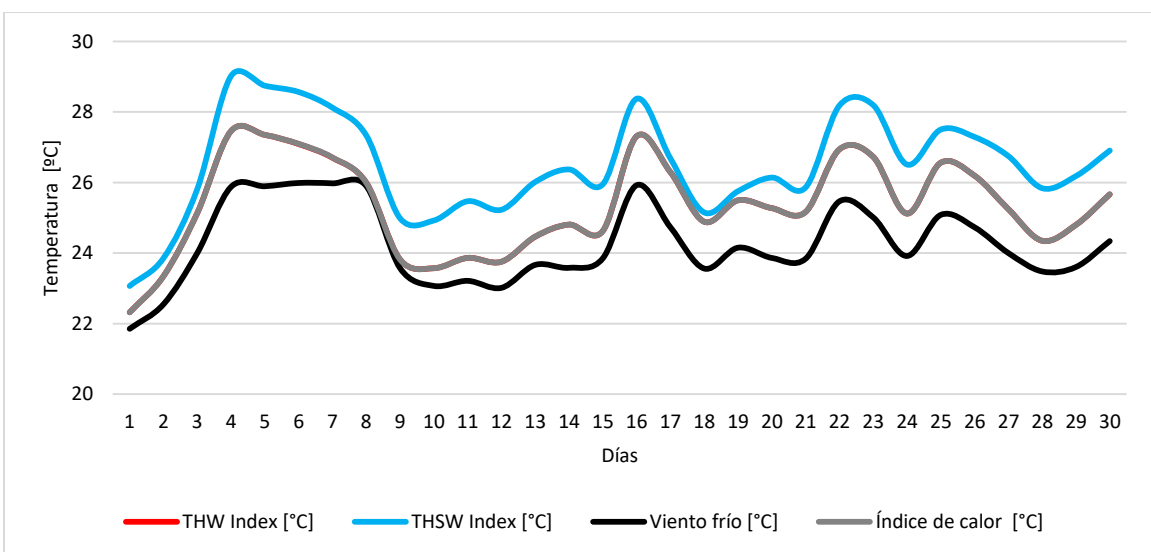
Figura 7. Índices de confort térmico. Abril de 2024
