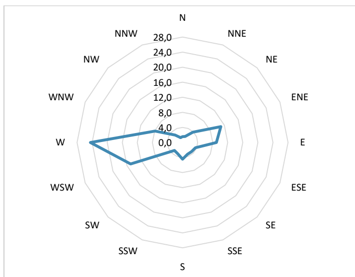
Figura 3. Dirección desde donde provienen los vientos. Noviembre de 2023
