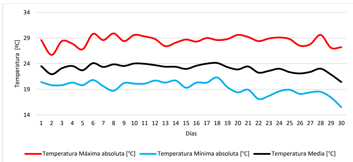
Figura 2. Temperatura del aire diaria (media, máxima y mínima). Noviembre de 2023
